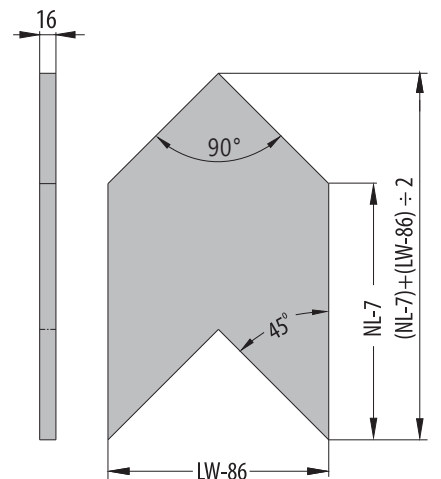
Wymiary dna Drawer bottom dimensions Размеры днища
